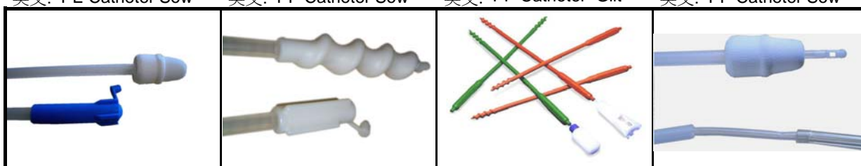
編號: 102.025 中文: PP授精棒(小球/藍尾塞) 英文: PP Catheter Gilt 編號: 103.021C 中文: 前端白螺旋授精棒 英文: Spirette catheter 編號: 103.022C 中文: 橡膠綠螺旋授精棒 英文: Melrose Catheter 規格: 編號: 104.200C 中文: 子母授精棒 英文: Foamtip catheter with inner cannula
